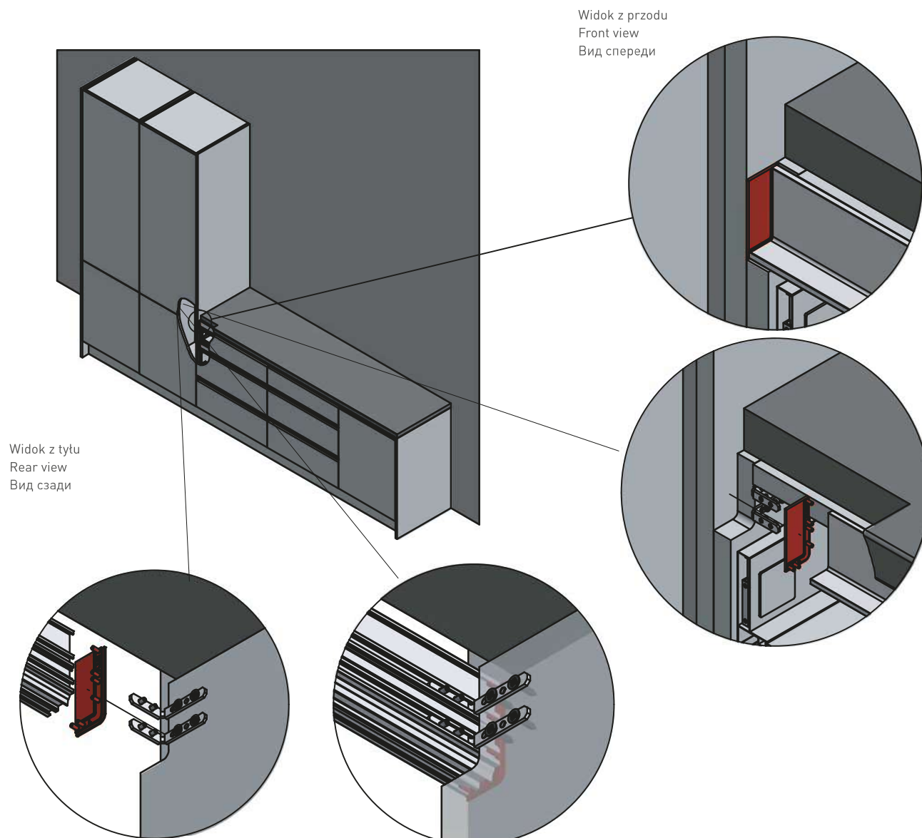
Przekrój boczny Side section Боковая секция
